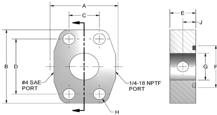
GAGE PORT SPACER- CODE61
